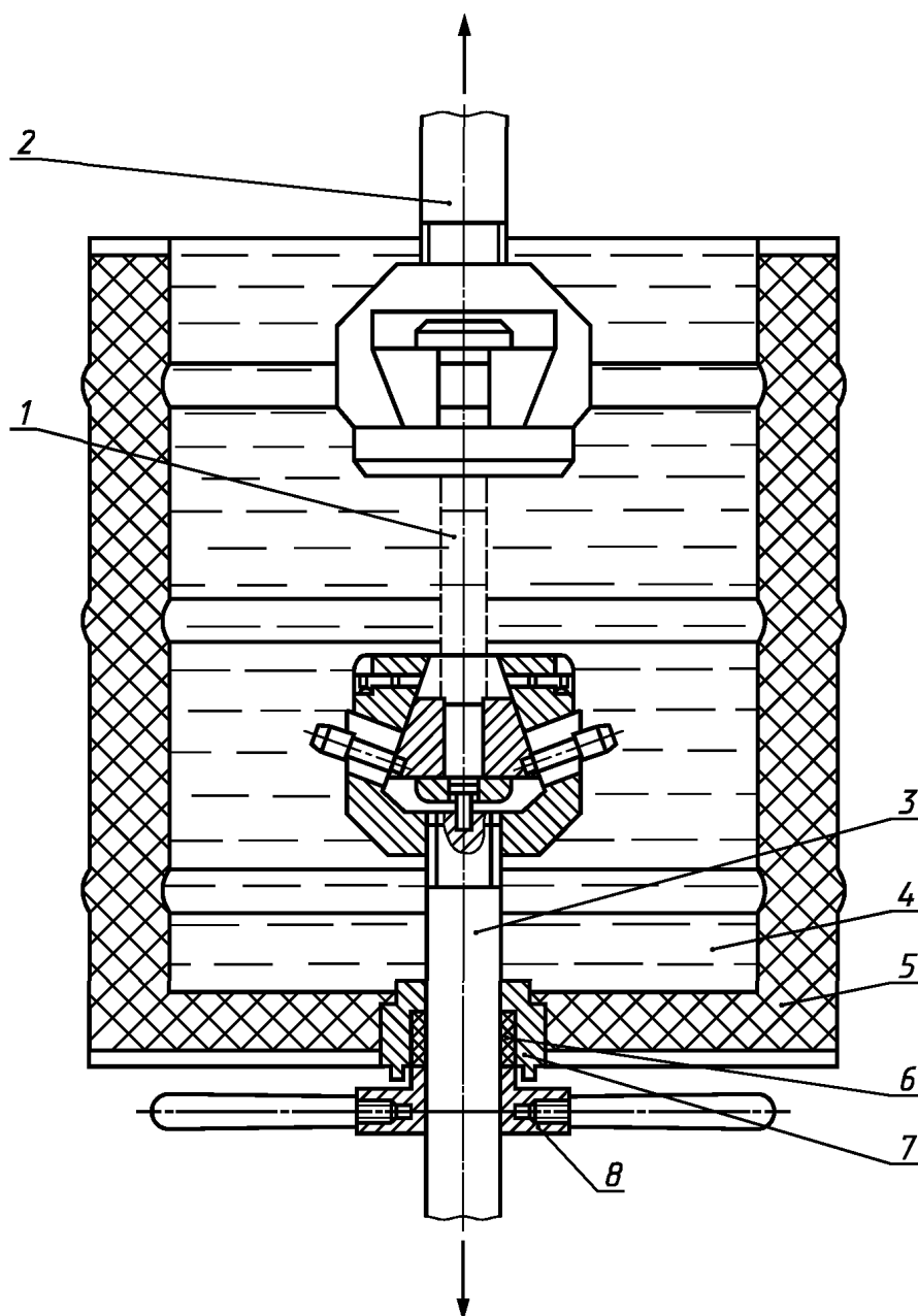
Схема размещения образцов в негерметизируемом криостате
