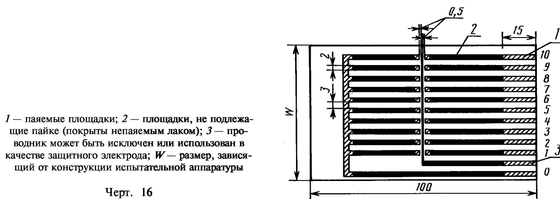
Подложка для механических и электрических испытаний
