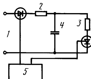
Тиристорная схема
