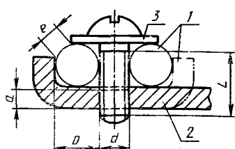
Винт, требующий шайбу или прижимную пластину
