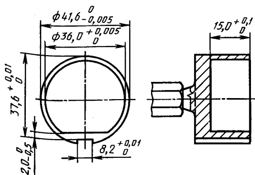
Калибр Б
