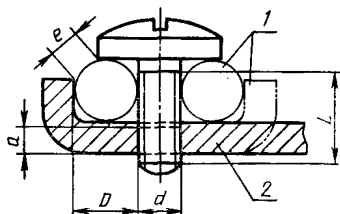
Винт, не требующий шайбы или прижимной пластины
