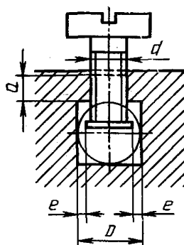
Зажим без прижимной пластины
