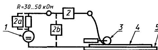
1 — источник напряжения 110 В; 2 — индикаторное и счетное устройство (2a и 2b — возможные расположения); 3 — роликовый электрод; 4 — испытуемый образец; 5 — плоский электрод
