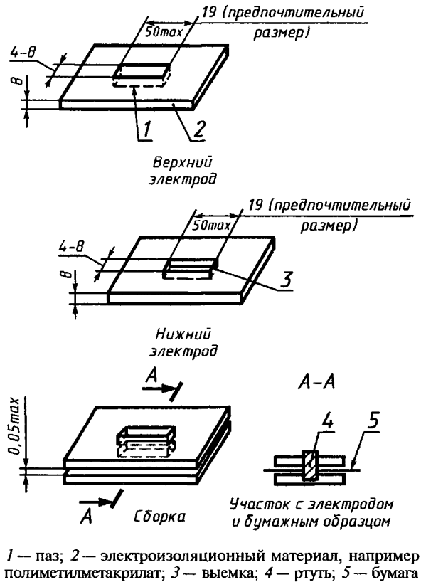
Рисунок 6 — Схема установки с ртутными электродами для определения проводящих включений методом 3
