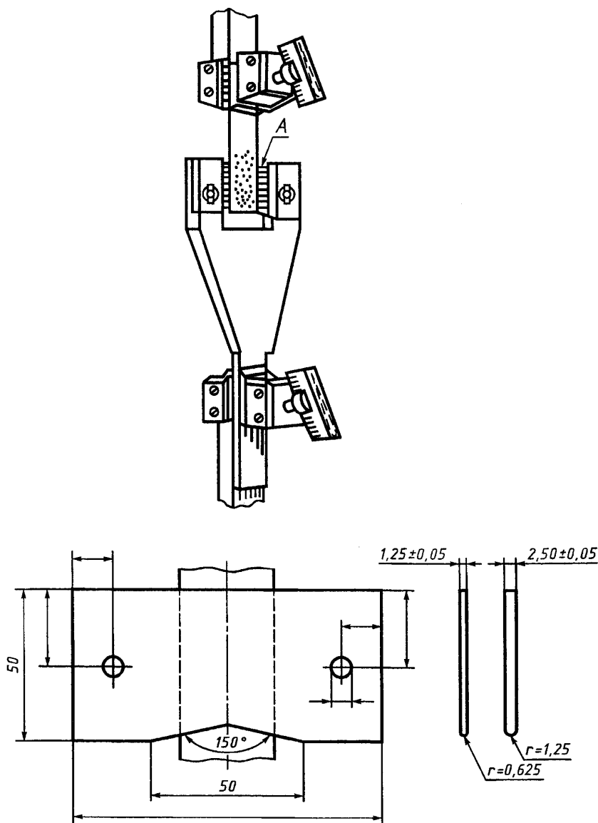
Рисунок 1 — Приспособление для надрыва кромки бумаги
