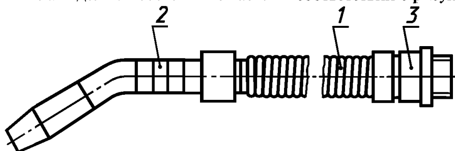
1 — рукав; 2 — наконечник; 3 — патрубок
