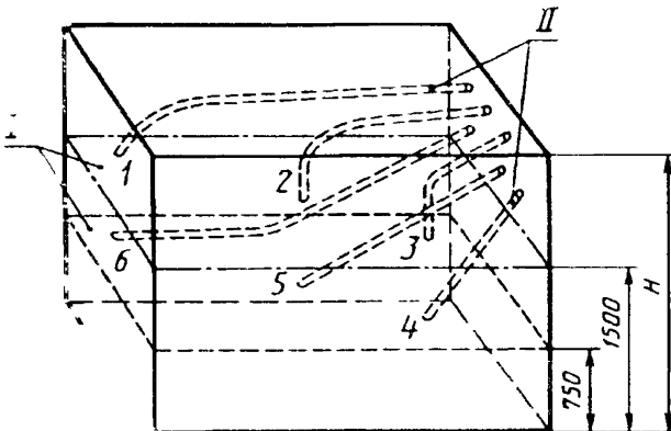
— уровни отбора проб воздуха (750, 1500 мм), II — трубки для отбора проб воздуха из камеры, 1, 2, 3, 4, 5, 6 — точки отбора проб воздуха
