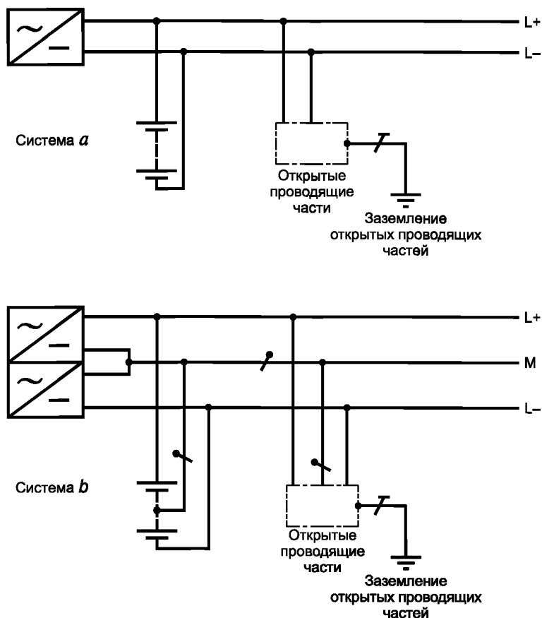
Рисунок 31К — Система IT постоянного тока
