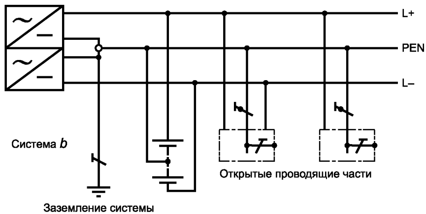
Рисунок 31G — Система TN-C постоянного тока
