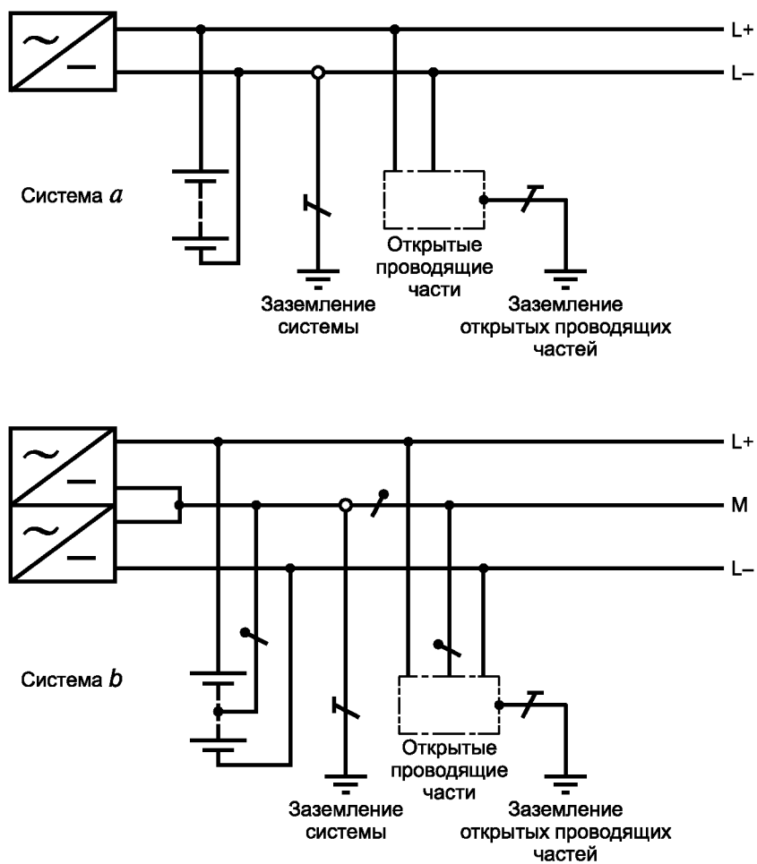
Рисунок 31J — Система ТТ постоянного тока
