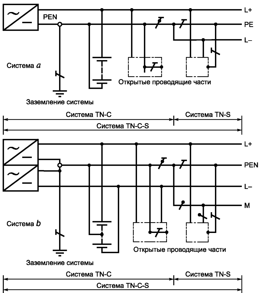
Рисунок 31Н — Система TN-C-S постоянного тока
