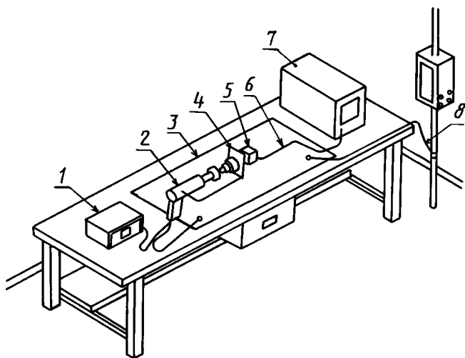
1 — источник питания; 2 — ИГ; 3 — плоскость заземления; 4 — мишень; 5 — аттенуатор; 6 — коаксиальный кабель; 7 — осциллограф; 8 — шины заземления
