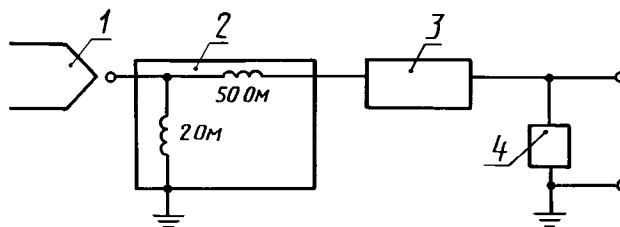
1 — ИГ; 2 — мишень; 3 — аттенуатор; 4 — осциллограф
