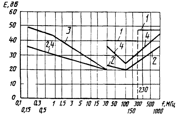
Нормы напряженности поля радиопомех
