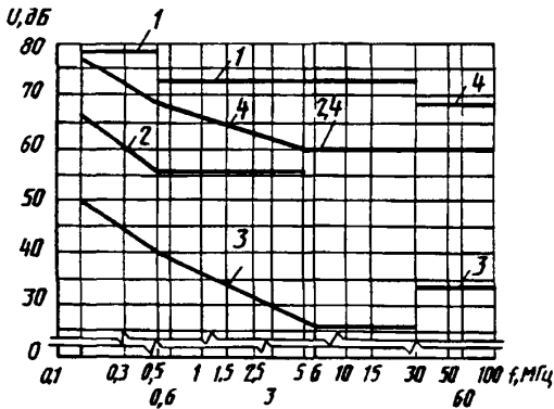
Нормы напряжения радиопомех
