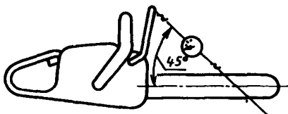
Рисунок 1 — Статическое испытание силы размыкания тормоза
