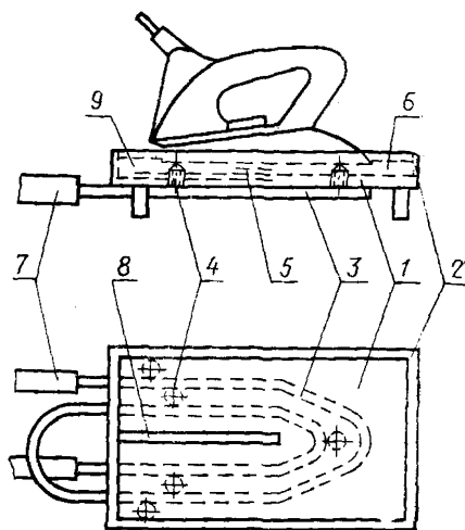
Прибор для проверки падения температуры подошвы утюга под нагрузкой
