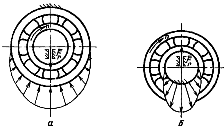
Виды нагружения (и эпюры нормальных напряжений на посадочных поверхностях)
