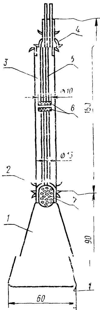
1—колба; 2—пробка; 3—стеклянный; 4—пробка; 5—кожух; 6—шлифт; 7—тампон; 8—трубчатый
