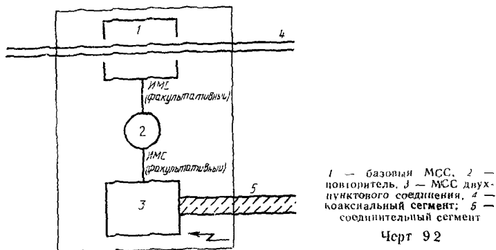
Повторительная установка, конфигурация коаксиал — соединение
