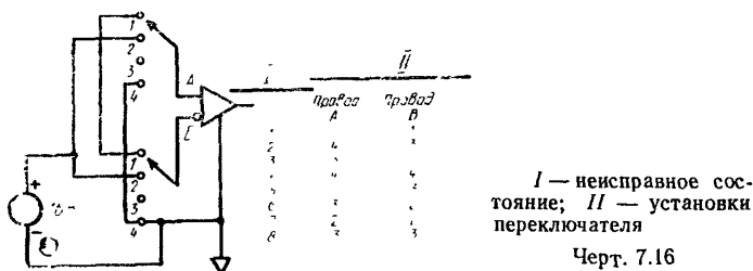
Неисправные состояния приемника
