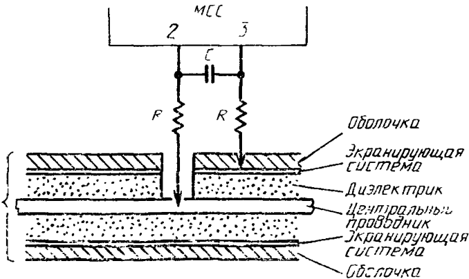
Типовая схема коаксиального ответвительного соединения
