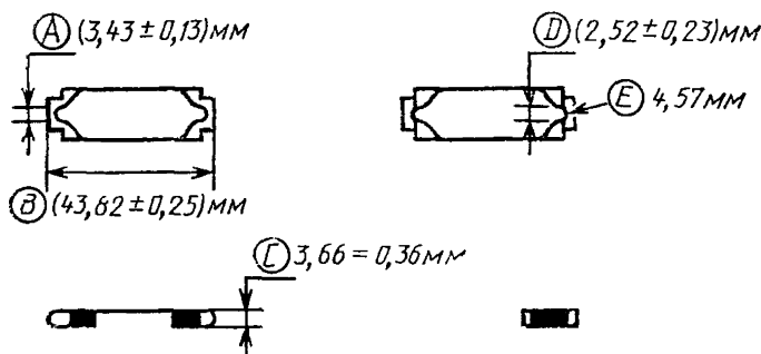
Скользящая защелка соединителя (максимальный размер материала 24)
