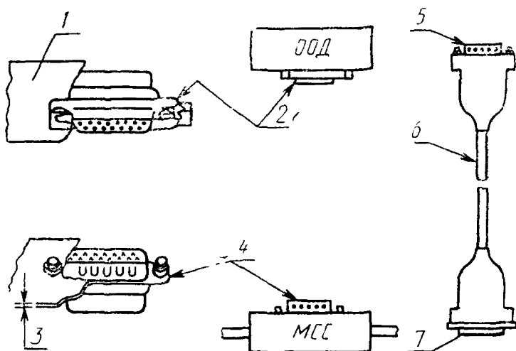
Детали соединителя и конфигурации кабеля ИМС
