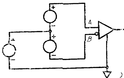
Проверка общего напряжения на входе приемника
