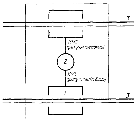
Повторительная установка, конфигурация коаксиал — коаксиал
