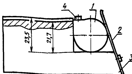
Приспособление для контроля размера 23,5—1,8
