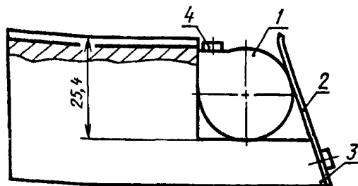
Приспособление для контроля размера 25,4 тах
