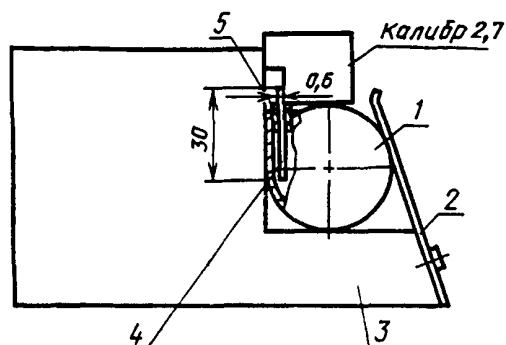
Приспособление для контроля размера 2,4 тах
