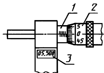
Цифровое устройство микрометров типов МВМЦ, МВТЦ, МВПЦ
