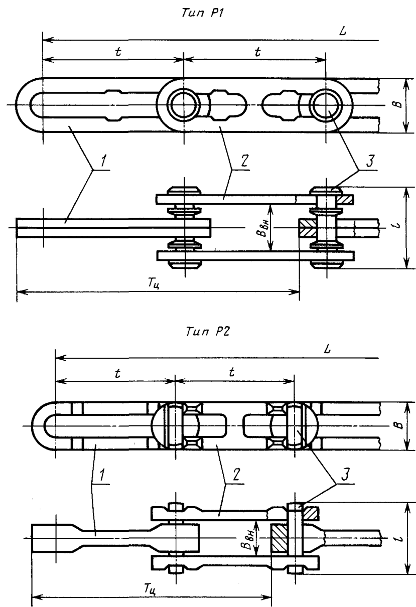
1 — внутреннее звено; 2 — наружное звено; 3 — валик
