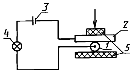
1 — образец; 2 — металлический брусок; 3 — источник питания; 4 — лампочка; 5 — пластинки
