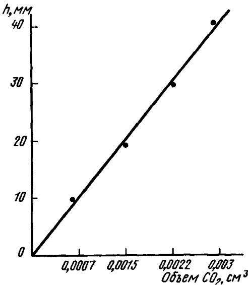
Градуировочный график хроматографа по двуокиси углерода
