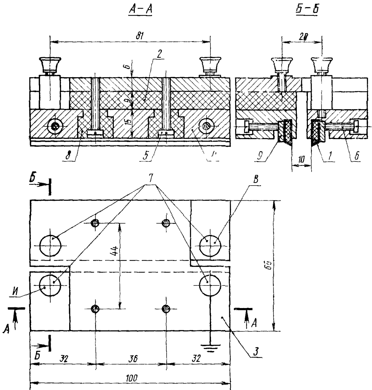
1 — ножевые электроды (резина, обернутая фольгой); 2 — прокладка; 3 — основание; 4 — электродные бруски; 5 — винты для крепления; 6 — прижимные винты; 7 — клеммы; 8 — втулки; 9 — планки прижимные, В — высоковольтный электрод; И — измерительный электрод.
