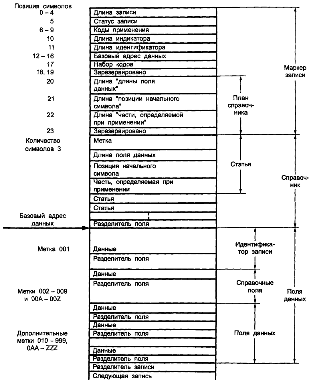
Рисунок 2 — Структура записи
