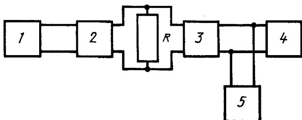
1 — испытуемый ТА; 2 — питающий комплект; 3 — селективный вольтметр; 4 — частотомер; 5 — электронный вольтметр переменного напряжения; R — резистор сопротивления (600 \pm 60) Ом, мощностью не менее 0,25 Вт
