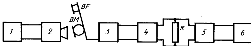
1 — генератор сигналов низкочастотный; 2 — искусственный рот; 3 — испытуемый ТА; 4 — питающий комплект; 5, 6 — измерители нелинейных искажений с ручной регулировкой; BF — телефон испытуемого ТА; BM — микрофон испытуемого ТА; R — резистор сопротивлением (600 \pm 60) Ом, мощностью не менее 0,25 Вт
