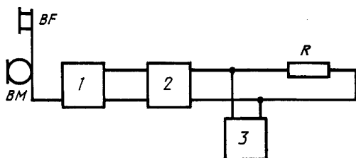
1 — испытуемый ТА; 2 — питающий комплект; 3 — измеритель электрических шумов (псифометр); R — резистор сопротивлением (600 \pm 60) Ом, P = 0,25 Вт; BM — микрофон испытуемого ТА; BF — телефон испытуемого ТА
