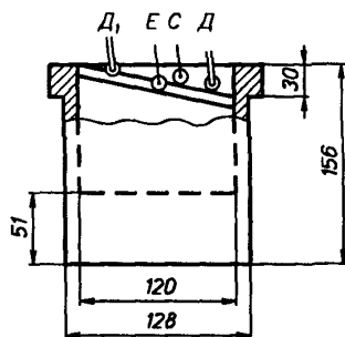
Рисунок 1 — Зональный пробоотборник
