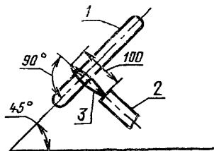
1—образец, 2—горелка, 3—пламя
