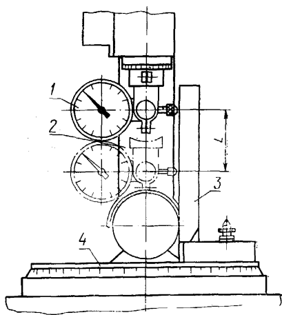
1 — индикатор; 2 — колонка микроскопа; 3 — угольник; 4 — предметное стекло
