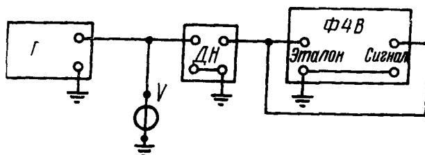
Γ—измерительный генератор; V—образцовый вольтметр; ДН—безреактивный делитель напряжения, Ф4В—поверяемый фазочувствительный вольтметр.
