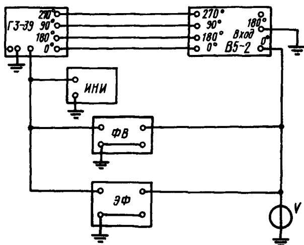
Схема поверки вольтметра В5—2
