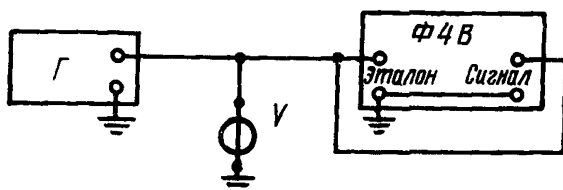
Γ—измерительный генератор; V—образцовый вольтметр; Ф4В—поверяемый фазочувствительный вольтметр.
