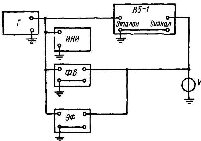
Схема поверки вольтметра В5—1
