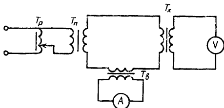
Схема размагничивания трансформатора тока
