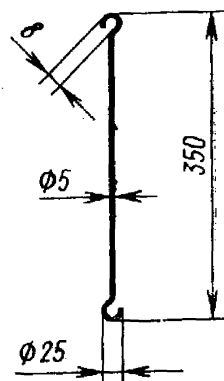
Удлинительная штанга
