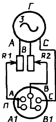
Г — генератор трехфазного напряжения; R1, R2 — переменные резисторы; П — проверяемый синхронскоп.
