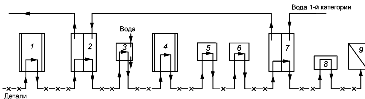
Рисунок 7 — Схема промывки деталей, покрываемых металлами, не способными к контактному выделению
