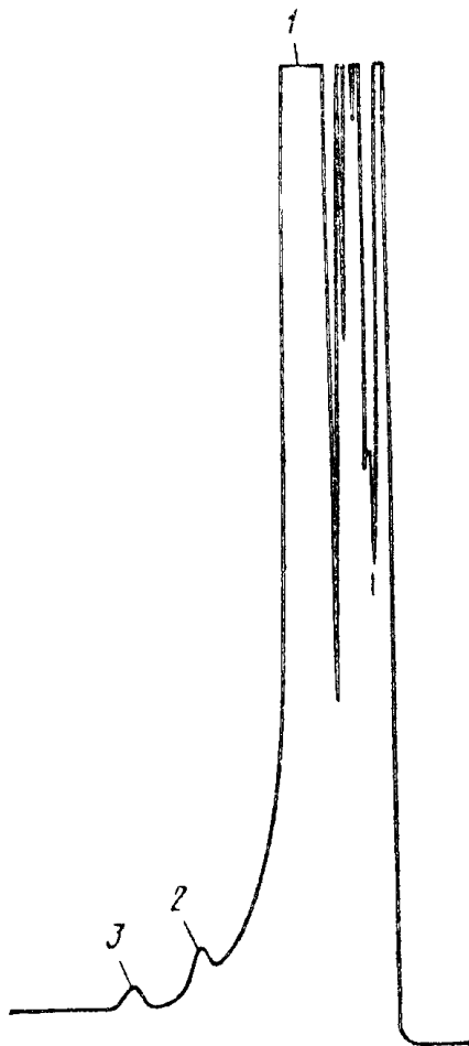
1—этилбензол; 2— p -цимол, 3—диэтилбензол
