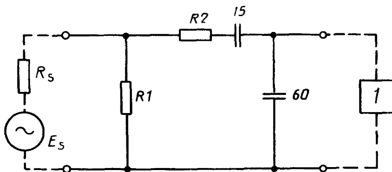
1 — радиоприемник, E_s — ЭДС источника сигнала; R_s — номинальное выходное сопротивление источника сигнала; R_1 — резистор сопротивлением, равным номинальному выходному сопротивлению источника сигнала, R_2 — резистор сопротивлением, определяемым из условия R_2 = (80 - \frac{R_s}{2}) Ом
