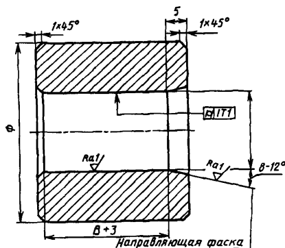
Рисунок 7 — Кольцевой калибр
