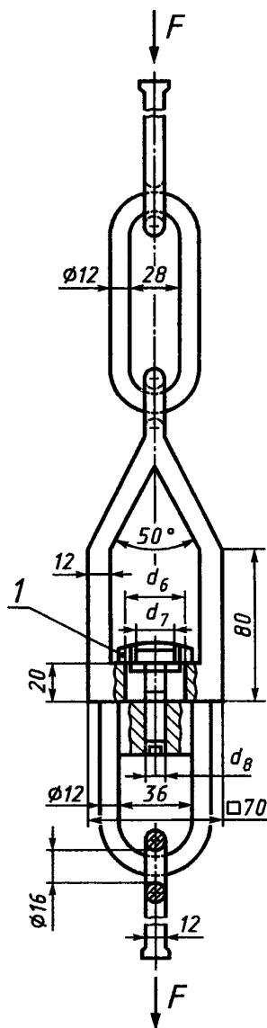
Рисунок 2 — Образец приспособления для испытания на растяжение Т
