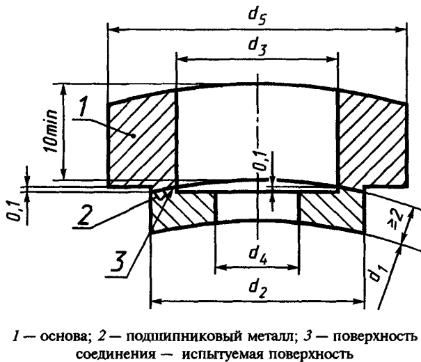
Рисунок 3 — Испытуемый образец (из радиального подшипника скольжения)
