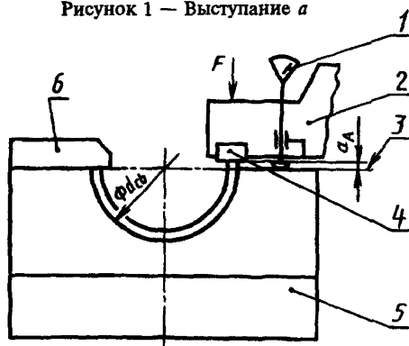
a_A — значение выступания
