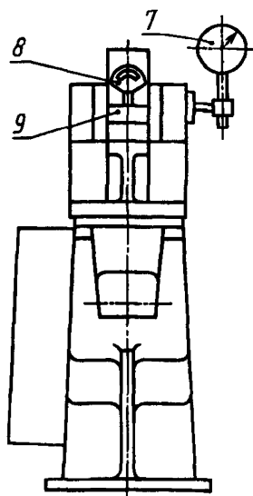
1 — самоустанавливающаяся опорная пята; 2 — контрольный блок; 3 — клапан регулирования давления; 4 — приводной двигатель; 5 — масляный насос; 6 — рабочий цилиндр; 7 — манометр; 8 — индикатор; 9 — подвижная измерительная головка
