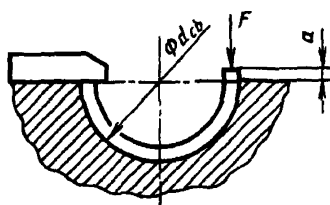
Рисунок 1 — Выступание a
