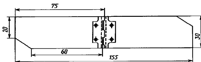
Рисунок 2 — Давильная пластинка
