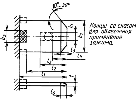
Рисунок 14 — Ответная часть зажима (лепесток), лист 1
