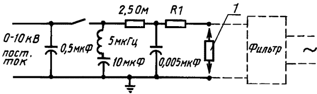
1 — испытуемый участок
