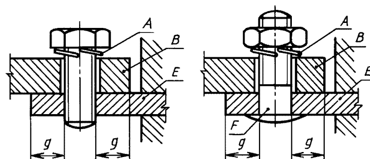
A — блокирующее устройство; B — наконечник или переключатель; E — закрепленная часть; F — штифт
