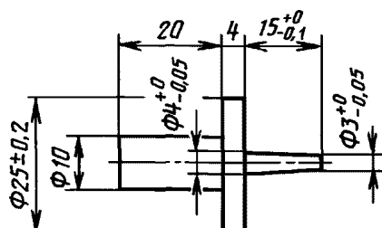
Рисунок 1 — Испытательный стержень
