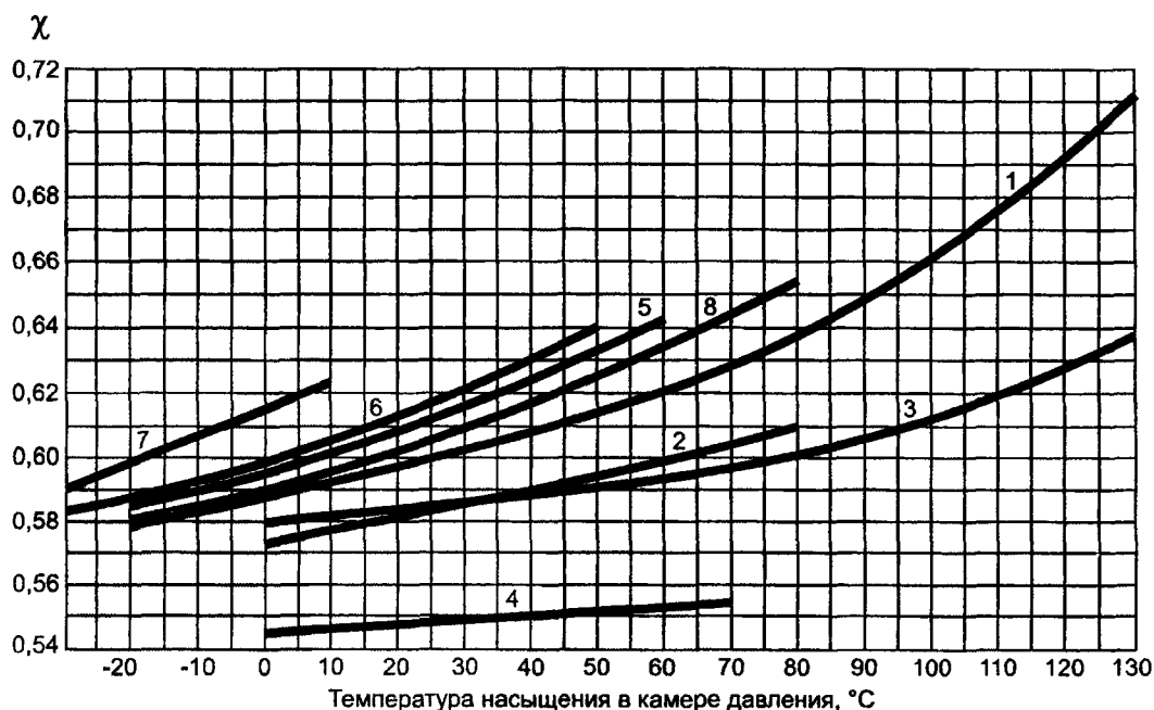
Рисунок Б.3 — Значение коэффициента \chi для критического давления потока.
