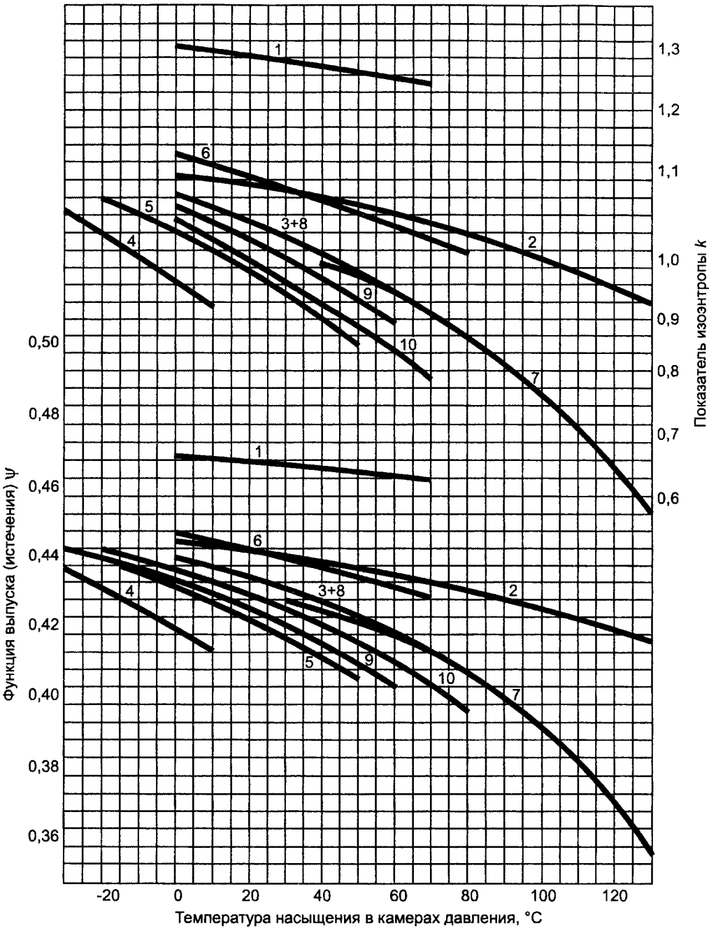
1 — R717; 2 — R11; 3 — R12; 4 — R13; 5 — R13B1; 6 — R22; 7 — R114; 8 — R500; 9 — R502; 10 — пропан
