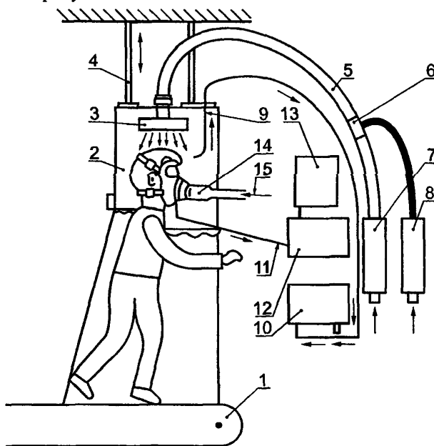
Рисунок 6 — Схема испытательной установки для определения коэффициента подсоса под полумаску/четвертьмаску с использованием гексафторида серы
