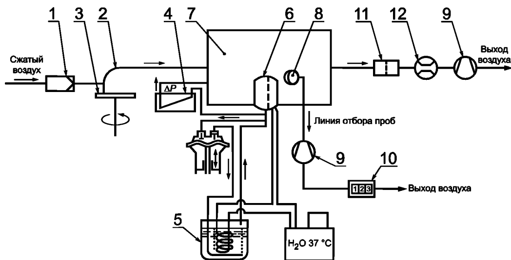
Рисунок 10 — Схема синусоидальной испытательной установки для определения устойчивости к запылению с использованием доломитовой пыли
