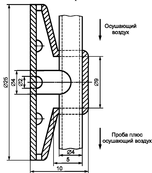
Рисунок 5 — Пробоотборник
