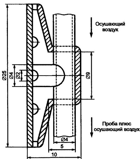
Рисунок 5 — Пробоотборник
