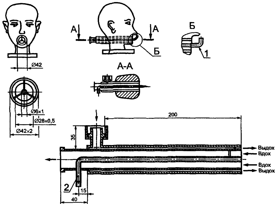
1 — втулка для измерения сопротивления воздушному потоку; 2 — измерение CO 2
