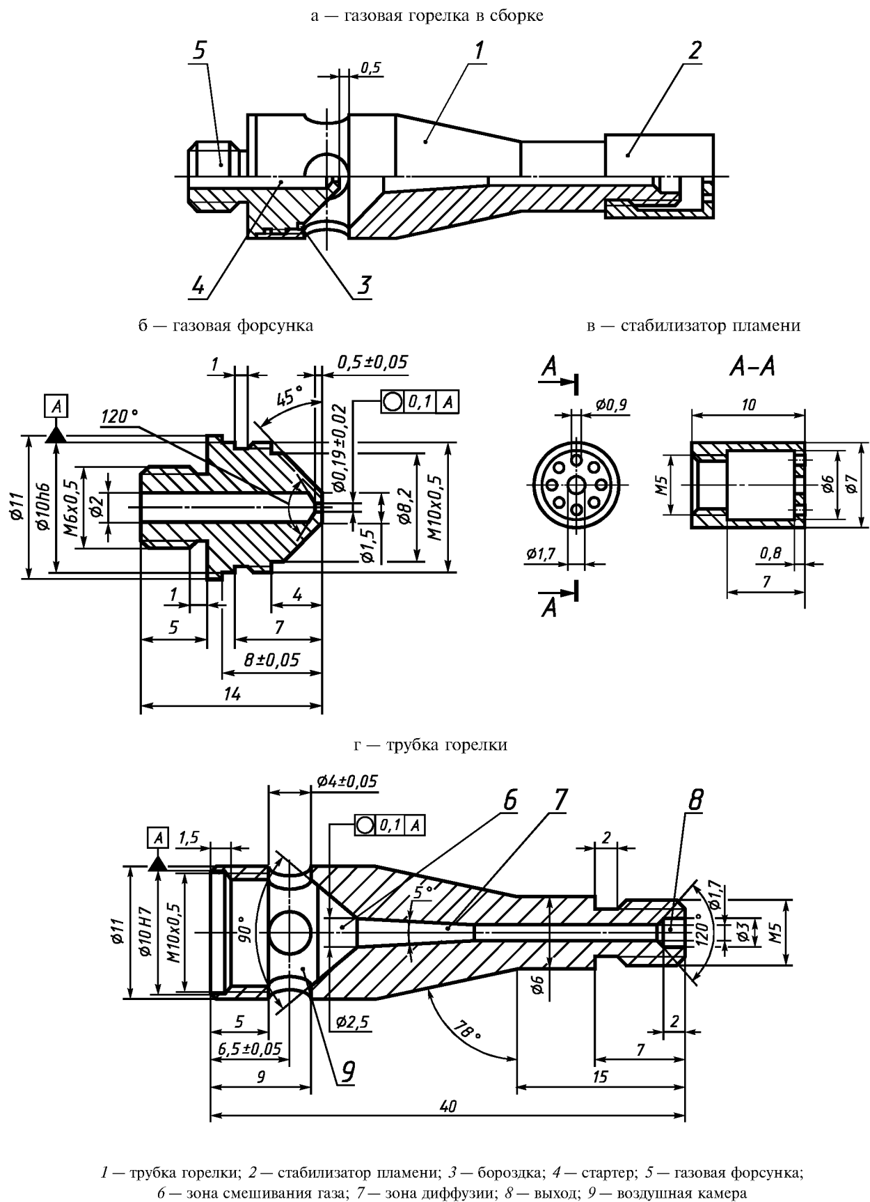
Рисунок 2 — Газовая горелка
