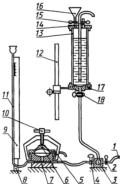
1 — спускная трубка; 2—4 — краны; 5 — трубина; 6 — крышка; 7 — основание; 8 — стойка; 9 — шкала давления; 10 — винт; 11 — трубка; 12 — штатив; 13 — стеклянный цилиндр; 14 и 15 — краны; 16 — воронка; 17 — держатель штатива; 18 — кран
