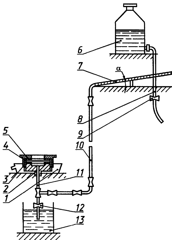
1 — ванна; 2 — полую камера; 3 — крышка; 4 — резиновая уплотняющая прокладка; 5 — металлическая прокладка; 6 — сосуд с тубусом для воды; 7 — стеклянная градуированная трубка; 8, 11 — резиновые трубки; 9, 12 — зажимы на трубках; 10 — стеклянная трубка; 13 — бачок для слива воды
