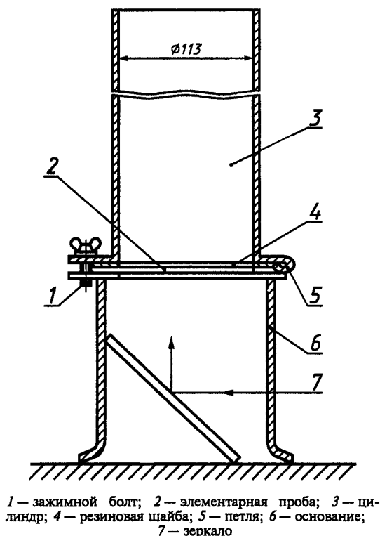
Рисунок 2 — Прибор для оценки водопроницаемости методом для низкого гидростатического постоянного давления
