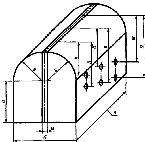
Испытательная конструкция 2
