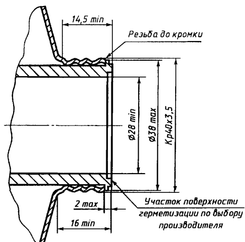
Рисунок 2 — Внешняя резьба с гnezдом САТ для крепления любого оборудования, кроме фильтров
