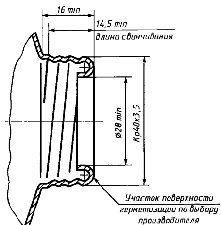
Рисунок 1 — Внешняя резьба без гnezда СА для фильтров
