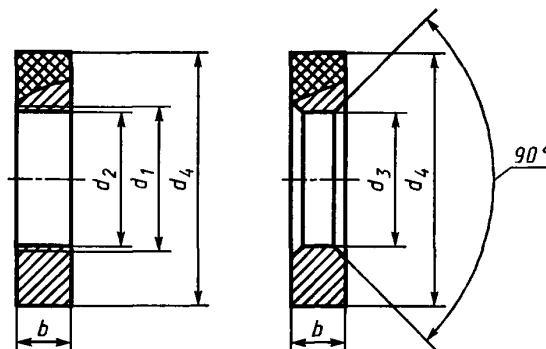
Проходной калибр
