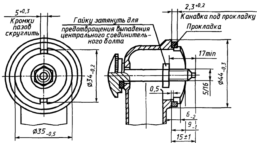
Рисунок 1 — Соединительное колено АА
