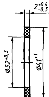
Рисунок 2 — Прокладка соединительного колена АА
