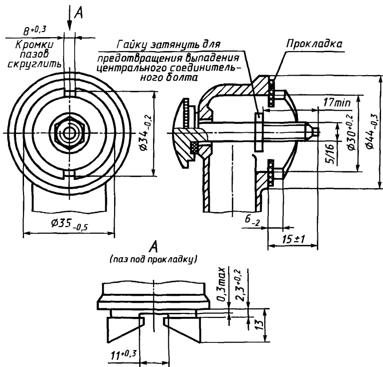
Рисунок 3 — Соединительное колено ВА
