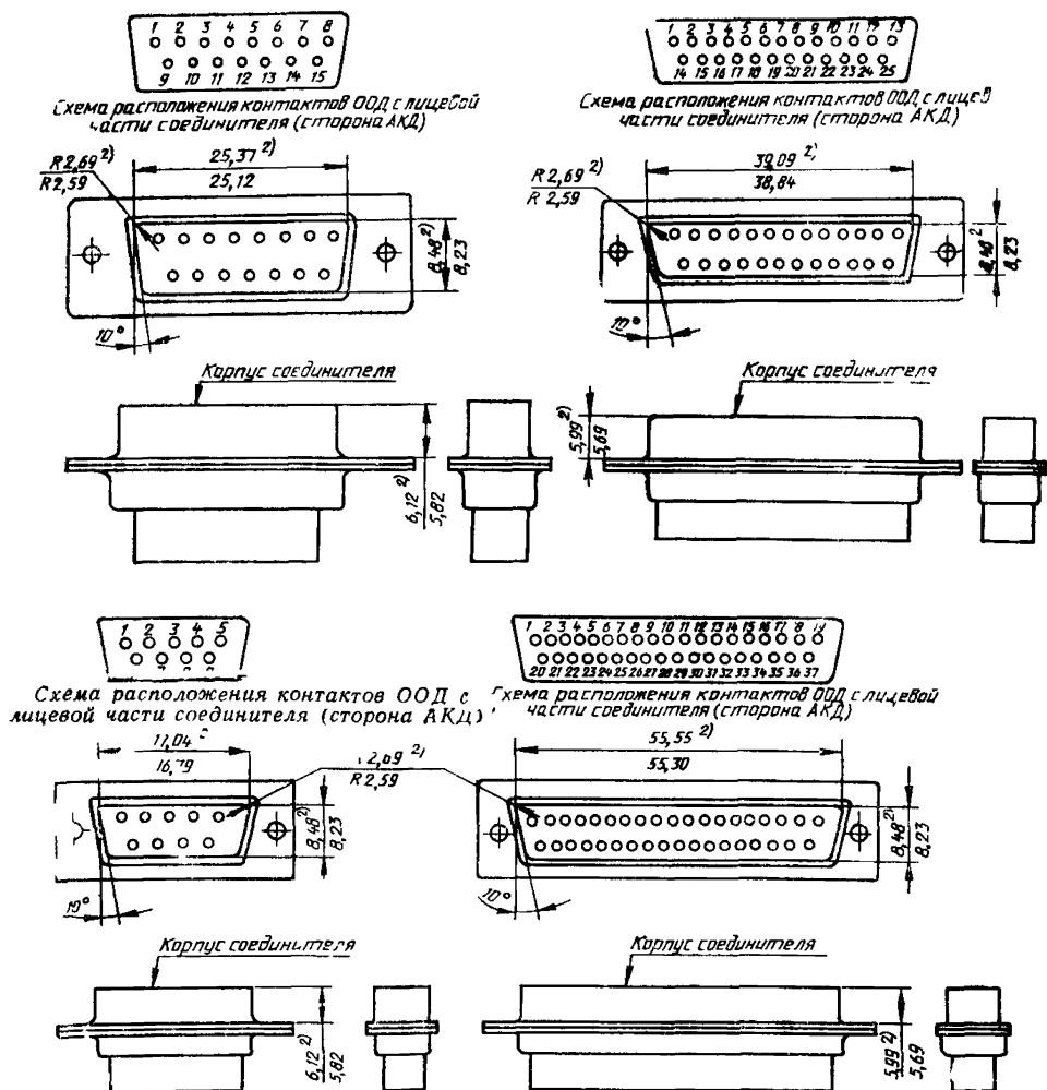
Рисунок 4.1 — Соединитель ООД
