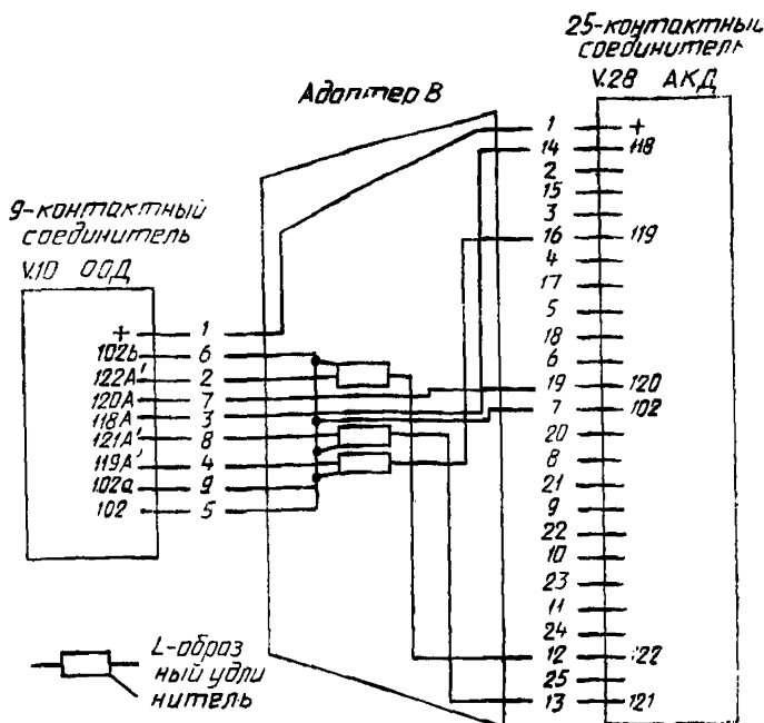
Рисунок G.5г. — 9/25-контактный базовый адаптер, конструкция В
