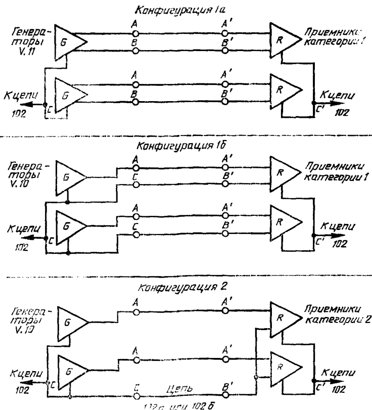
Рисунок Е.1 — Конфигурации взаимосоединений генератор/приемник
