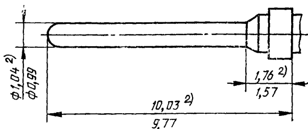
Рисунок 4.4 — Штыревой контакт
