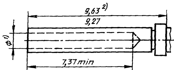
Рисунок 4.4 — Штыревой контакт
