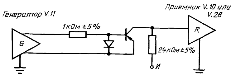
Рисунок D.1 — L-образный удлиннитель для защиты приемн V.10 или V.28
