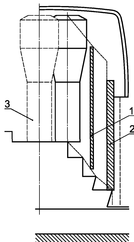
1 — щит; 2 — двойной щит; 3 — цилиндрическая фигура
