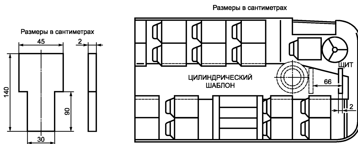
Рисунок 3.12 (см. 5.7.5.3.1)
