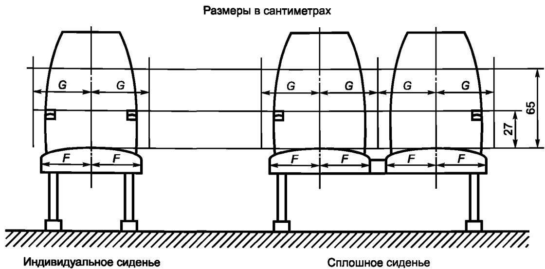
Рисунок 3.5 — Ширина пассажирских сидений (см. 5.7.9.1)
