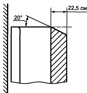
Рисунок 3.15 — Пространство для ног пассажира
