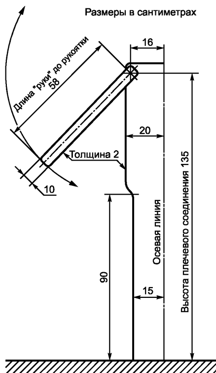
Рисунок 5.1
