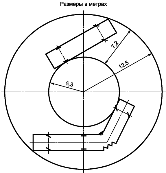
Рисунок 4.А
