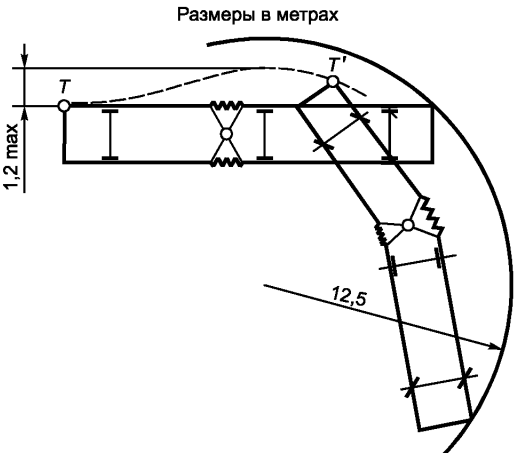
Рисунок 4.С
