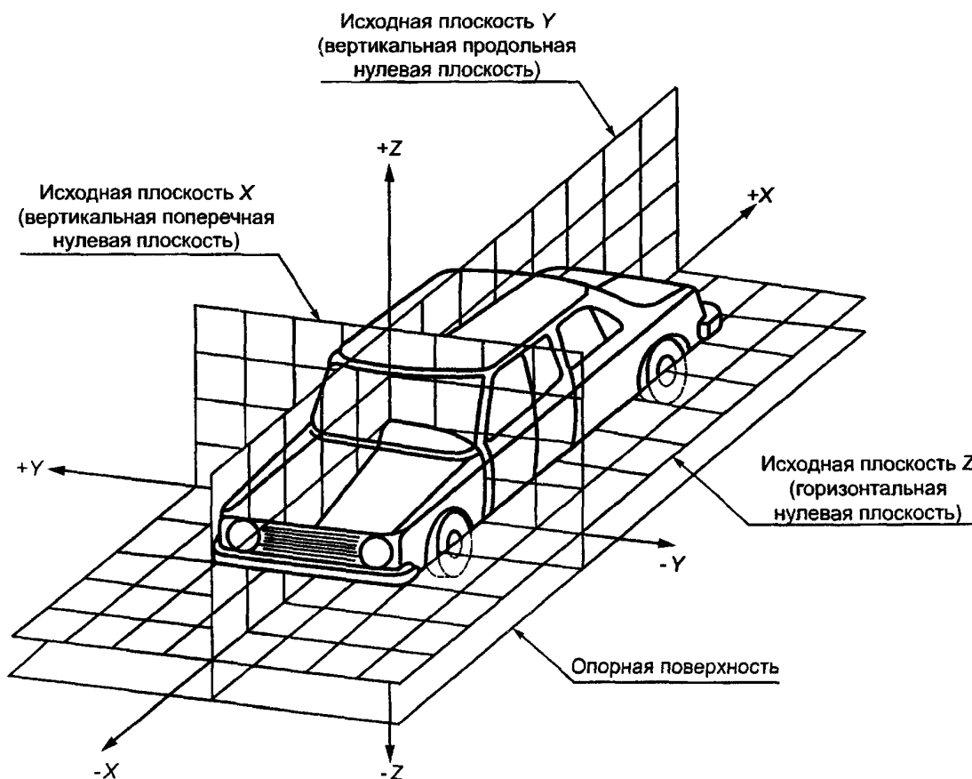
Рисунок 7.3 — Трехмерная система координат
