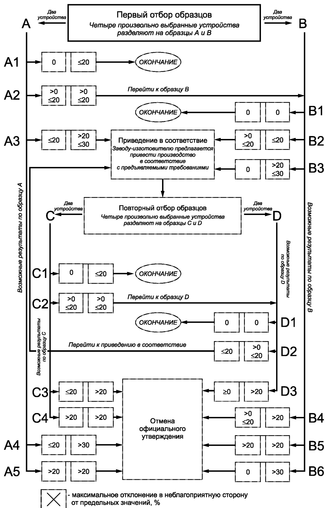
Рисунок 1 — Схема проведения процедуры отбора образцов
