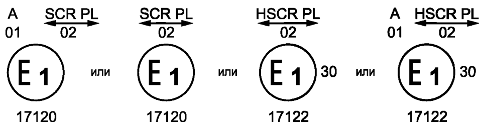
Рисунок 9 — Лампа, совмещенная с элементом HSB. Лист 1
