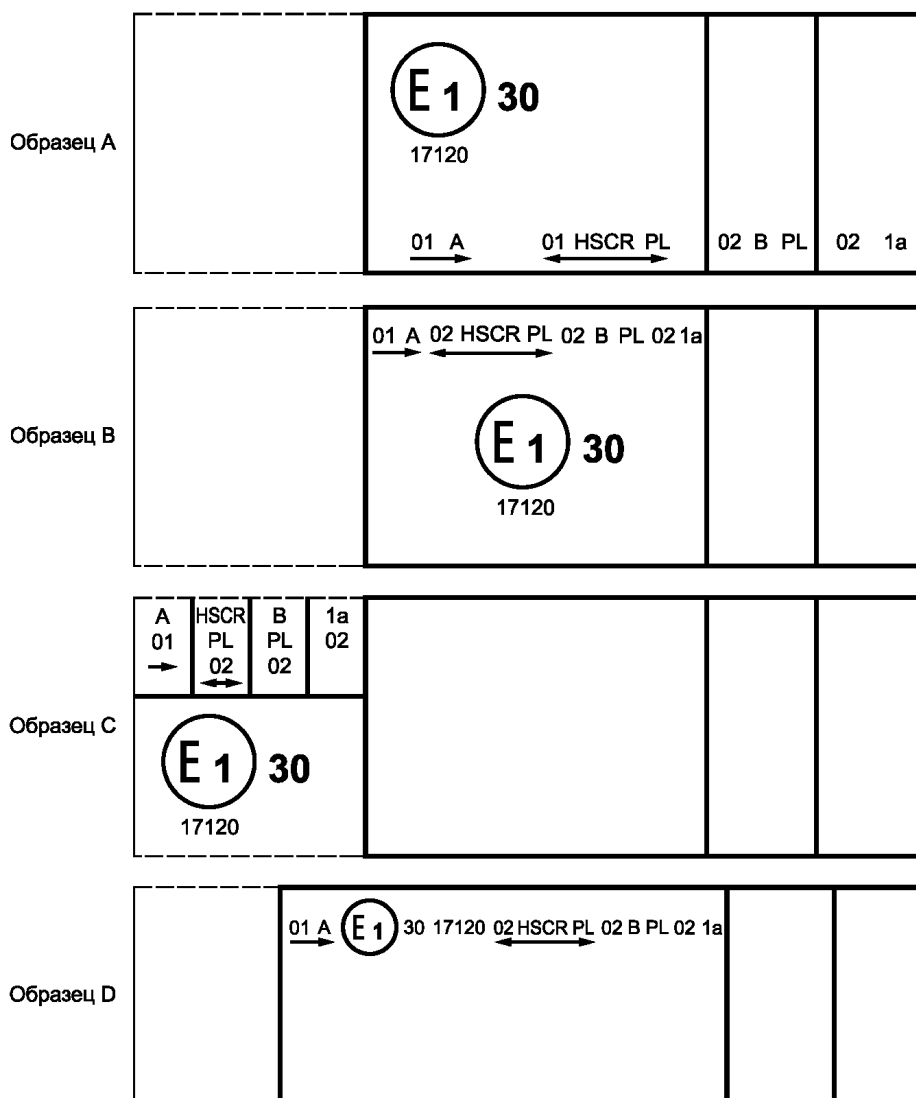
Рисунок 8 — Упрощенная маркировка сгруппированных, комбинированных или совмещенных огней
